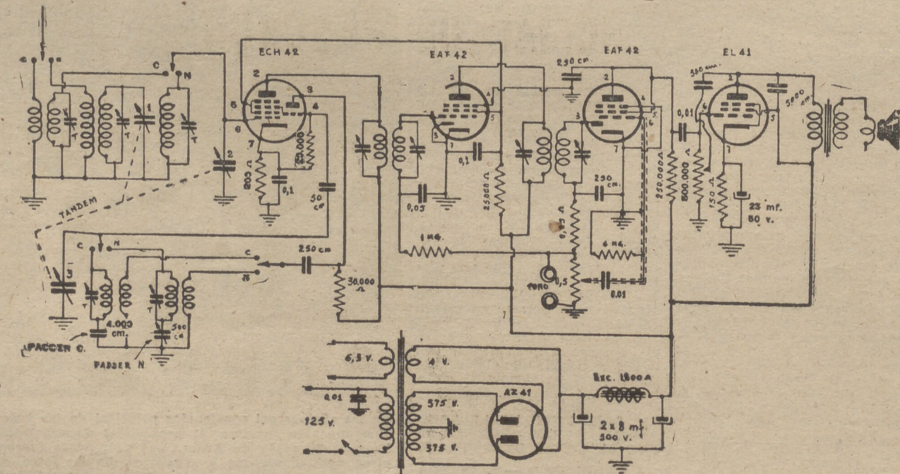
Fig. 142.—Circuito teórico del receptor proyectado
