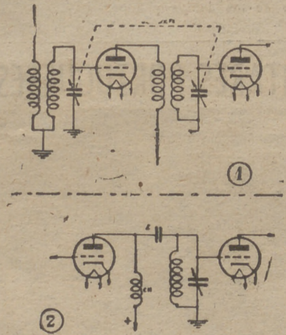
Fig. 84.—Acoplamiento de circuitos amplificadores en A. F.
