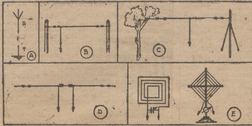
Fig. 3.—Símbolo y diversos tipos de antenas.
