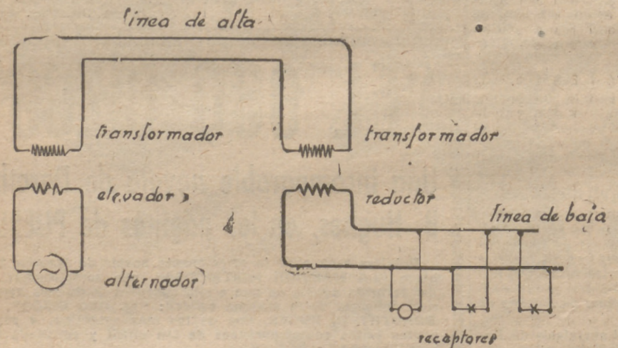
Esquema de una distribución monofásica
