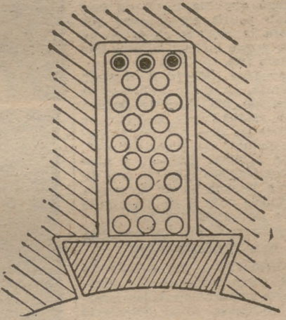
Ranura y bobina cortada con la tira de fibra de sujeción.
