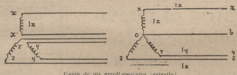
Unión de los arrollamientos (estrella)
