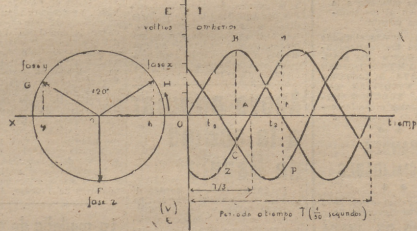
Representación gráfica de la corriente trifásica
