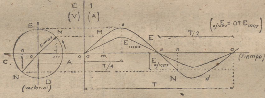
Representación gráfica de la corriente alterna
