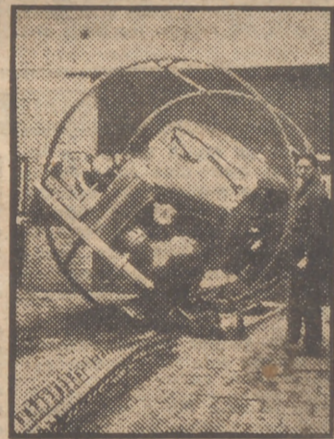
Por medio de este aparato, inventado por el holandés J. J. Neuteboom, el coche puede ser inspeccionado para su reparación en todos los sentidos. En pocos segundos, el automóvil da una vuelta completa. En cualquier posición puede mantenerse para los trabajos de reparación. (Foto A. P.)
