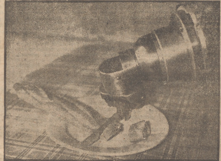
He aquí el aparato ortopédico inventado por M. François Garcin. Presenta el aspecto de una gran dinamo. Dotado de un brazo de acero, termina en una mano metálica. Puede realizar todos los movimientos del brazo humano. (Foto Cifra.)
