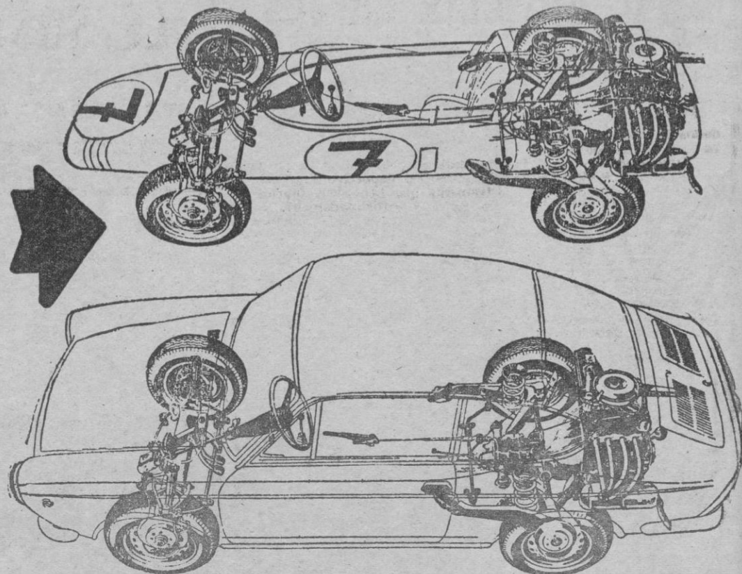
Como confirmación de lo mucho que la industria del automóvil obtiene de las experiencias proporcionadas por las competiciones, obsérvese este dibujo, en cuya parte superior se inserta un simil de lo que sería la mecánica del Seat 350 Sport Coupé con una carrocería de un vehículo de fórmula, y abajo lo que es el modelo normal. Desprovisto de la carrocería de serie, el automóvil posee características similares a las que definen los fórmulas: motor trasero longitudinal, salida de gases por colectores independientes, equipo eléctrico con alternador, refrigeración forzada de aceite, suspensión de ruedas independientes, frenos de disco delanteros, neumáticos de gran batón, etcétera.
