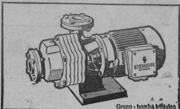
Grupo - bomba trifásico
