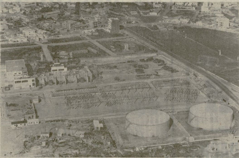
La nueva Central Térmica que Gesa ha construido en San Juan de Dios y que será inaugurada el próximo martes por el Ministro de Industria D. Gregorio López Bravo. Esta Central resuelve el problema de suministro eléctrico a Mallorca de forma definitiva. (LEA INFORMACION EN PAGINAS INTERIORES.)
