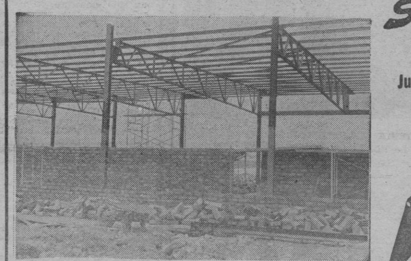
ESTRUCTURA METALICA PARA EDIFICIO EN EL AEROPUERTO DE SON SAN JUAN.
