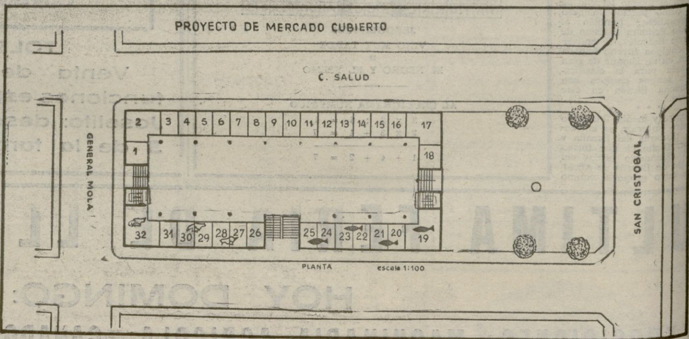
PLANO DEL MERCADO CUBIERTO, QUE MUY PRONTO VA A SER CONSTRUIDO EN EL ARENAL.
