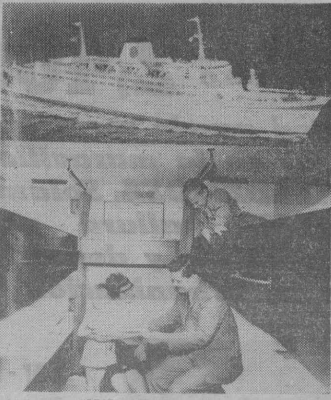
MAGNIFICO ASPECTO DEL TRANSBORDADOR SUECO «SAGA», GEMELO DEL BUQUE QUE HARA LA TRAVESIA BILBAO-SOUTHAMPTON. — 2) CONFORTABLE ASPECTO DE UN CAMAROTE DEL BUQUE — (Foto Citra)
