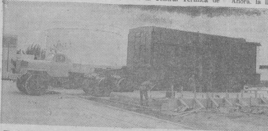
EL IMPONENTE CAMION —EL MAS GRANDE de MALLORCA— A PUNTO DE DEPOSITAR UNO DE LOS CUERPOS DEL GENERADOR DE 14.000 KWS. SOBRE LA PLATAFORMA QUE SE ESTA CONSTRUYENDO AL EFECTO Y QUE PUEDE APRECIARSE EN PRIMER PLANO
