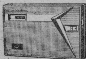
SAMOS
