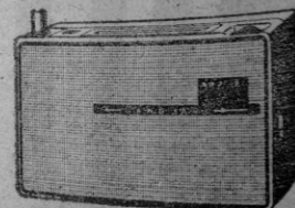
SUPER POLARIS
