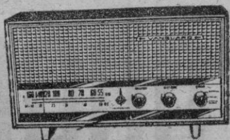
TIROS
