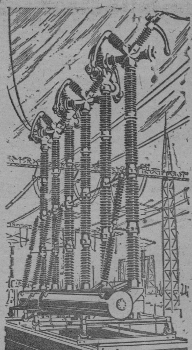
Primer interruptor de 420.000 Voltios y 20 millones kVA, de potencia disruptiva, puesto en marcha en febrero de 1962.
