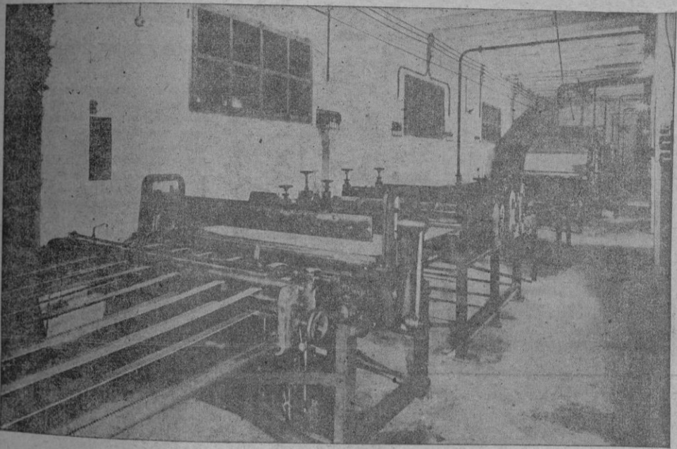
PERSPECTIVA DE LA SECCION PARA PLANCHA DE CARTON ONDULADO
