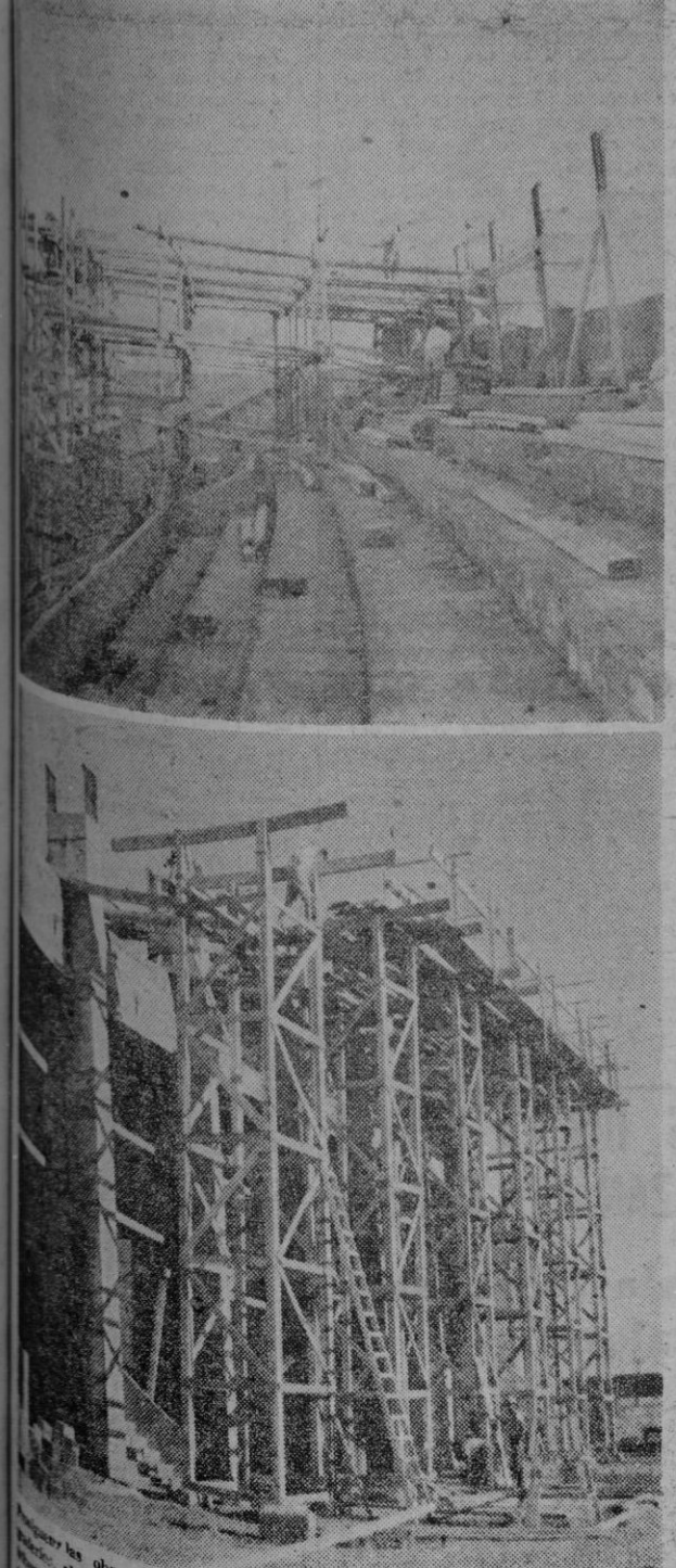
Las obras en el Estadio Balear. Una vez terminados todos los trabajos se procede a la construcción del alero que ha de cubrir la tribuna de preferencia. En las dos fotos de «Juanet» se pueden apreciar los andamios del andamio sobre el cual ha de apoyarse el techo de la mencionada tribuna.
