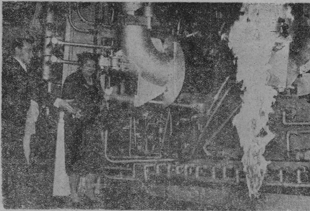
En Avilés, la esposa del Presidente del Instituto Nacional de Industria, doña Joaquina Mercader de Suances, aplica la lanza metálica con una antorcha encendida en el extremo, en la tobera número 19 del horno, quedando así encendido y puesto en servicio el segundo horno, llamado «Joaquina», en situación de producir mil setecientas toneladas diarias de lingote de hierro.
