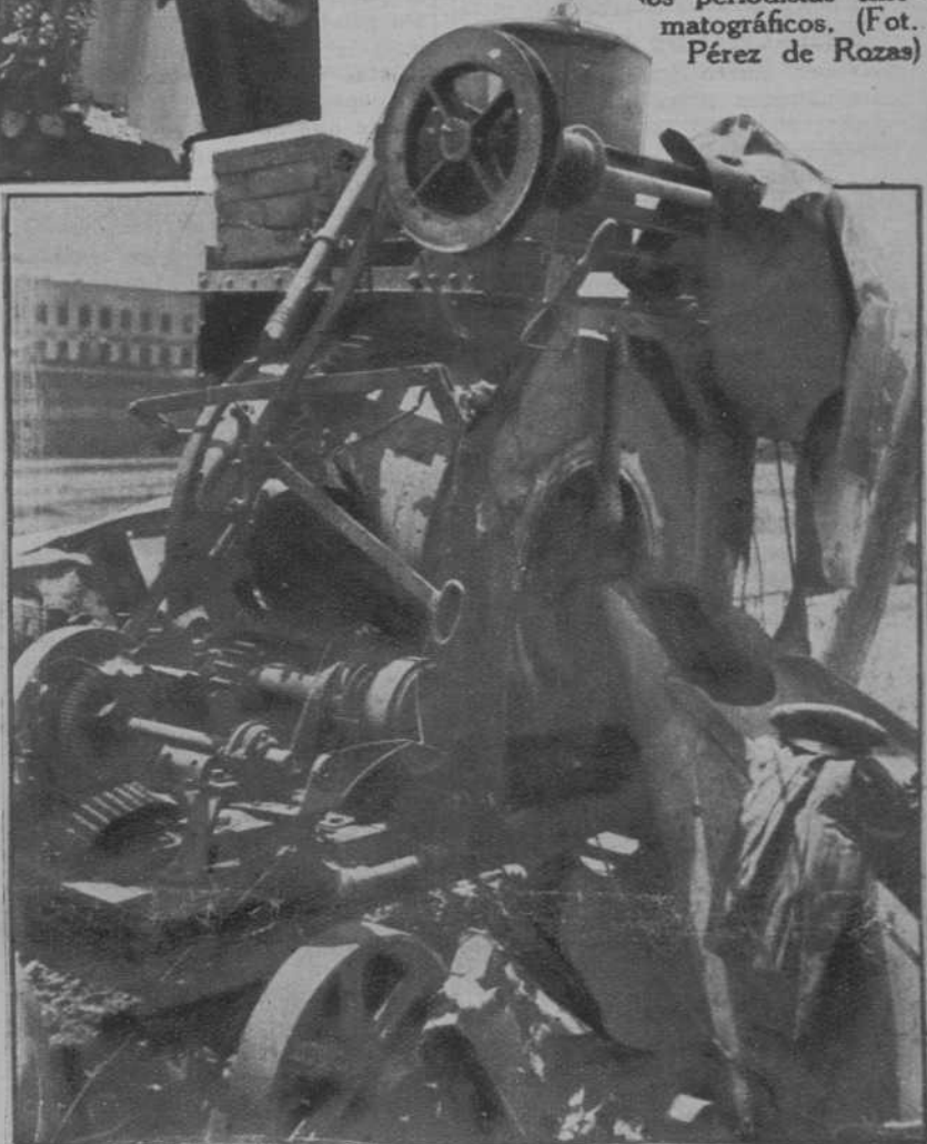
La trituradora de grava instalada en la calle de Provenza, frente a la estación de Sans, que fué destrozada la noche del domingo a causa de la explosión de una bomba (Fot. Pérez de Rozas)
