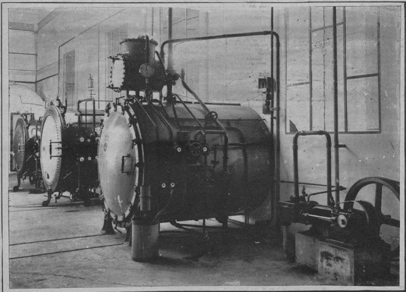
Bomba neumática y grandes autoclaves para la desinfección de ropas, en uno de los centros de desinfección del Instituto Municipal de Higiene
