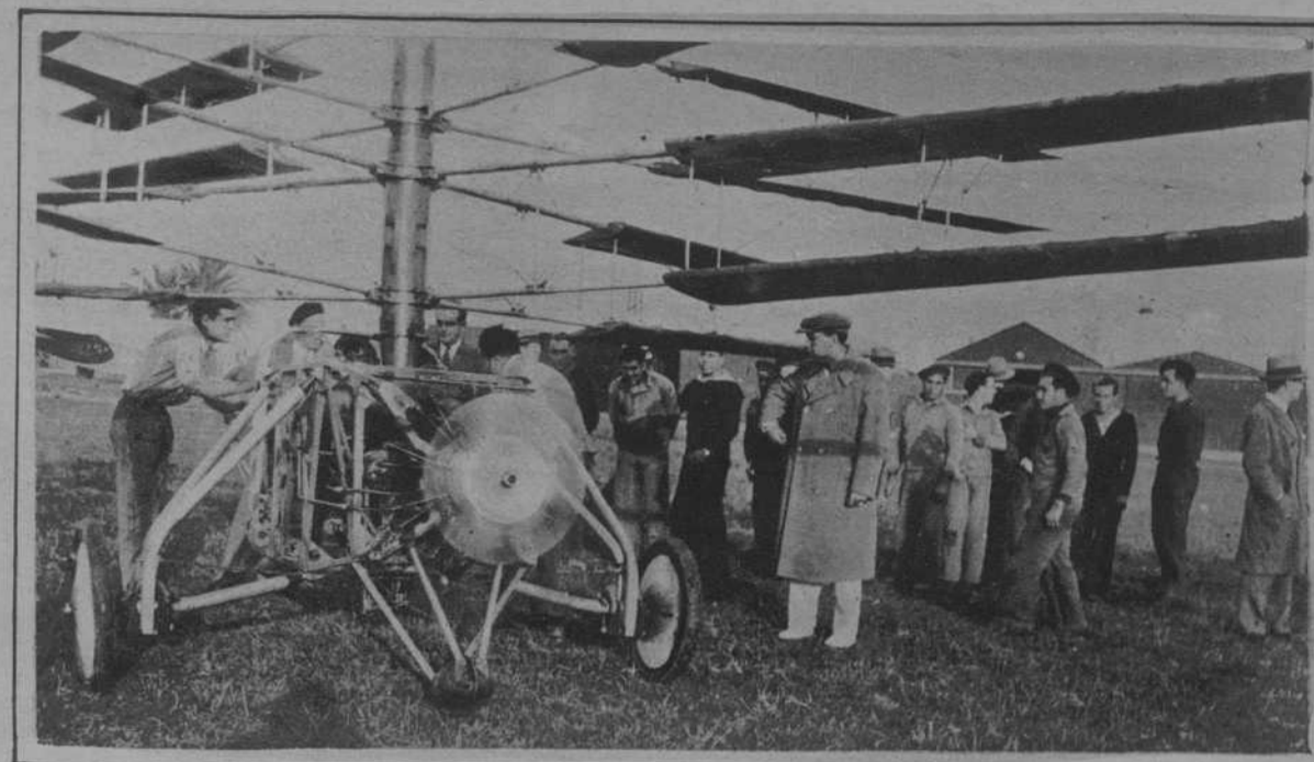
En el Aerodromo del Prat han tenido lugar las pruebas del helicóptero del marqués de Pescara, las cuales dieron buen resultado. — El marqués de Pescara dando instrucciones para los ensayos del helicóptero
