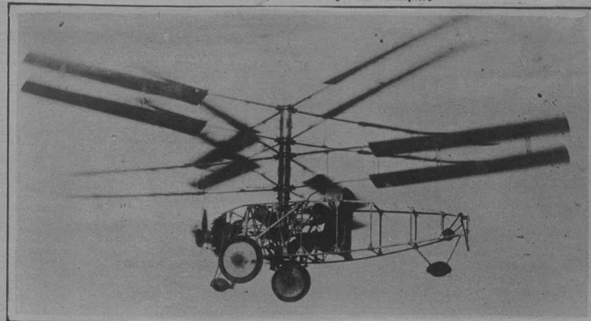
El helicóptero del marqués de Pescara, en pleno vuelo, pilotado por el señor Barrera. — (Fots. Merletti)
