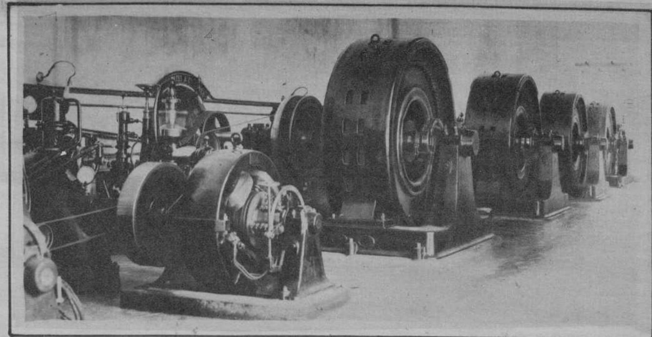
Sala de Maquinas de la Central hidroeléctrica de «La Pea»
