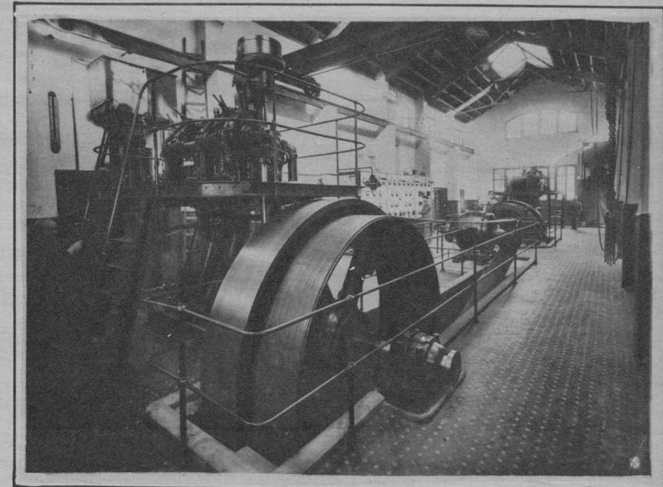
CENTRAL TERMICA DE JATIVA DE LA «UNION ELECTRICA LEVANTINA» Dos grupos Diesel Krupp, de 400 K. V. A.
