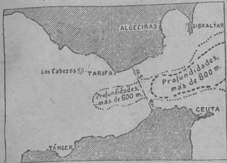
EL ESTRECHO DE GIBRALTAR Y SU ZONA DE GRANDES PROFUNDIDADES ENTRE ALGECIRAS Y CEUTA
