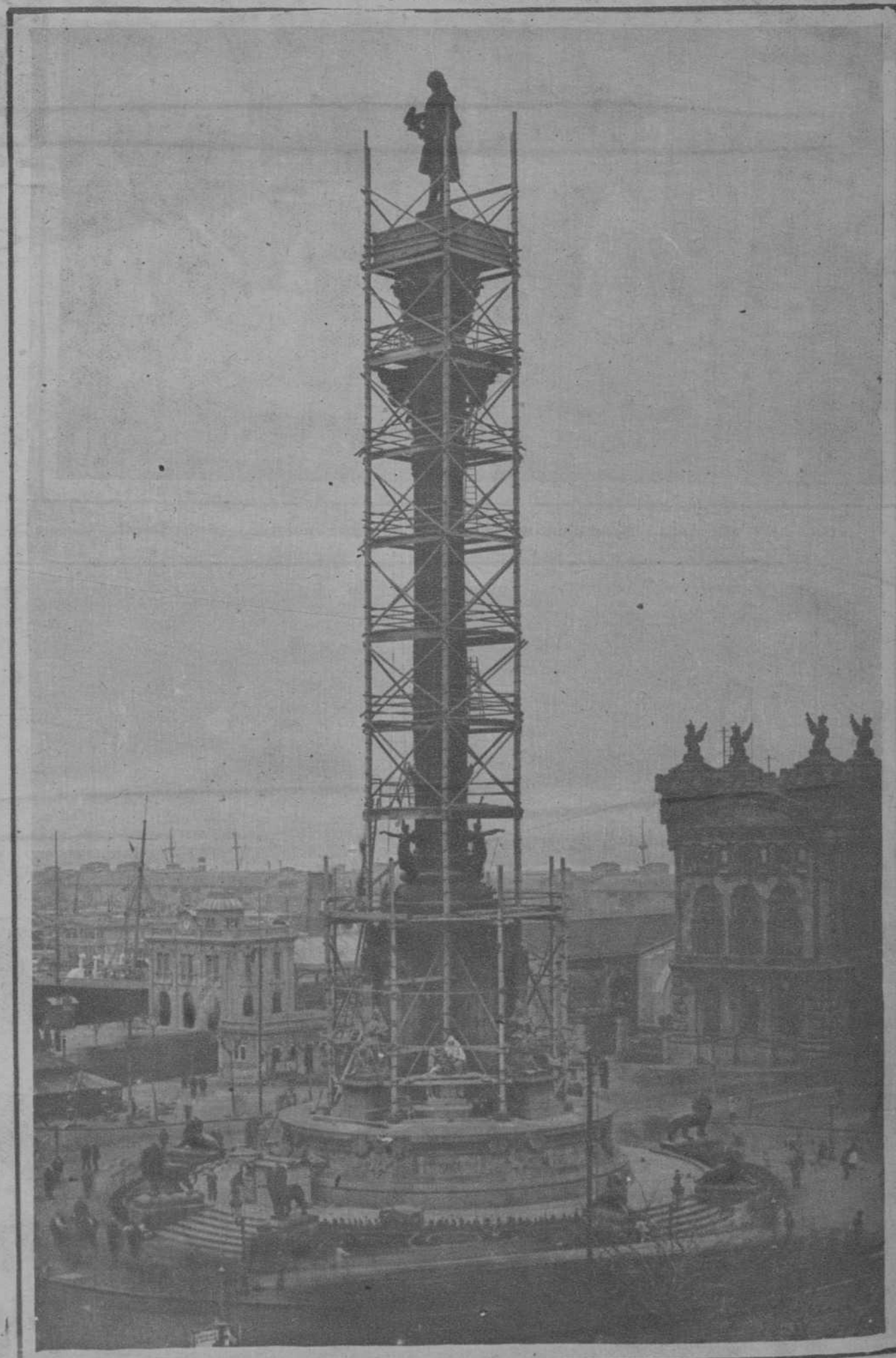
BARCELONA.—Atrevido andamiaje construido para la reparación del Monumento a Colón.—(Fot. Maymó)
