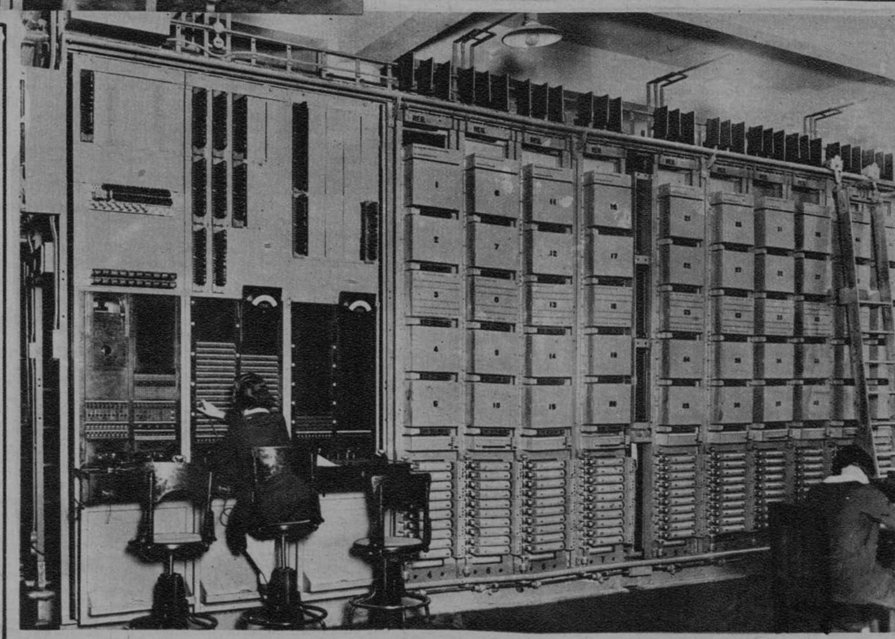
La mesa de telefonemas de la Central Automática ya en funciones. Esta es una de las secciones, 07, a donde los señores abonados pueden llamar desde su domicilio, sin necesidad de molestarse en ir a las Oficinas de la Compañía
