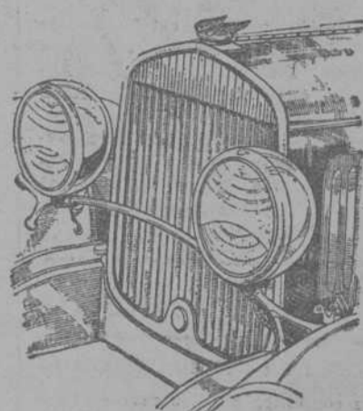
El radiador del Chrysler «75» con las persianas reguladoras de la temperatura del motor.
