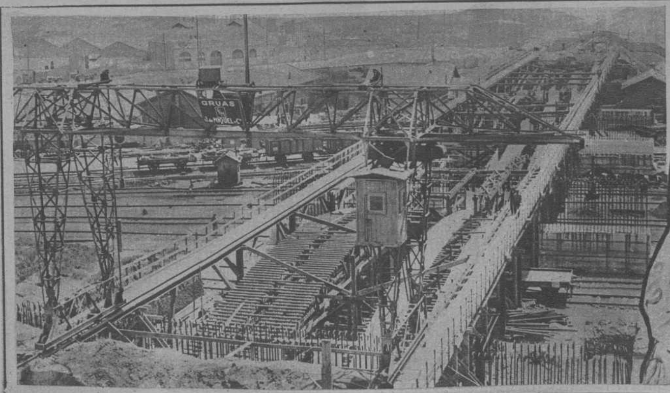
BARCELONA.—Estado de las obras en construcción del Viaducto de la calle de Marina, mejora urbana de gran importancia, realizada por la Comisión de Ensanche del Ayuntamiento barcelonés.
