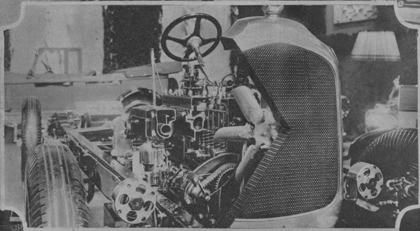
Corte longitudinal de uno de los soberbios Chassis Chrysler, que se adjudican la admiración de los inteligentes. (Fot. Badosa).
