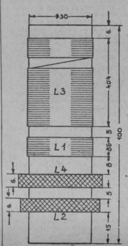
Detalles técnicos del esquema Tungsram de cuatro válvulas
