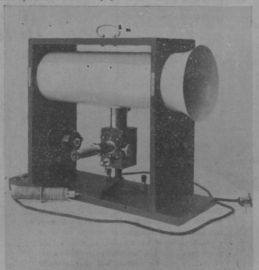
Aparato Gerdien, para determinar la conductibilidad eléctrica del aire
