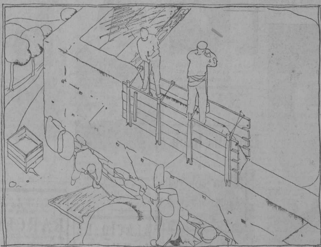
Esquema demostrativo de la técnica del tapial. Cinco hombres constituyen una cuadrilla de trabajo para cada tablero. Dos son apisonadores, otro amasador y dos peones (cavadores). Su rapidez es característica. Puede calcularse que ejecutan ocho metros cúbicos en la jornada de ocho horas
