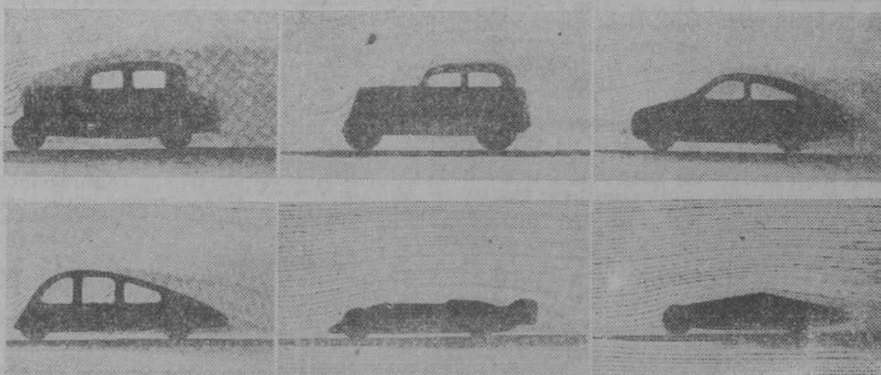
Ensayos por inyección de líquidos coloreados. Contrastan los torbellinos que corresponden a las formas ordinarias, con las penetraciones uniformes de las carrocerías aerodinámicas
