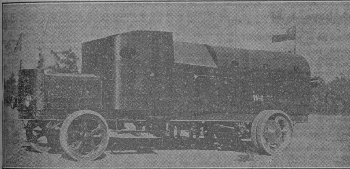
La República de Chile sigue sumida en convulsiones políticas de carácter bélico. Su Ejército se ha provisto de camiones blindados con que atender a los revoltosos. Aquí mostramos el camión White número 6 de cinco toneladas, provisto de un fuerte blindaje protector y armado con un cañón Krupp de 75 mm en la parte trasera y ametralladoras a cada lado.
