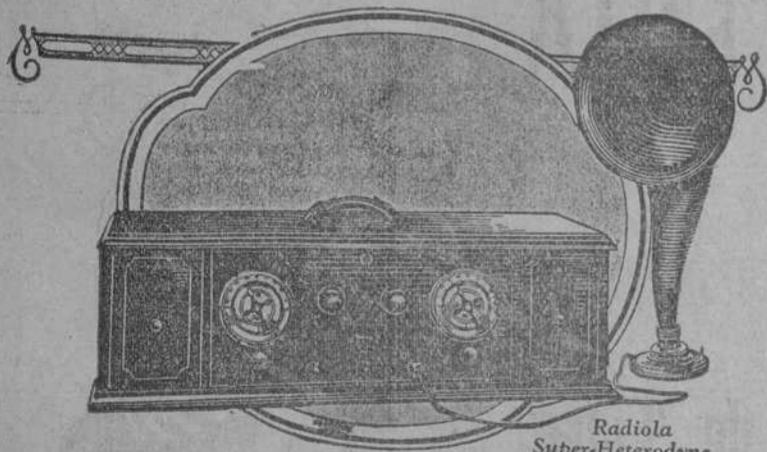
Radiola Super-Heterodyne. La caja, hermosamente acabada, se ha proyectado para dar cabida en su interior a todas las baterías. No requiere antena exterior ni conexión a tierra. Se suministra con seis Radiotrons UV-109 y Radiola Altoparlante.
