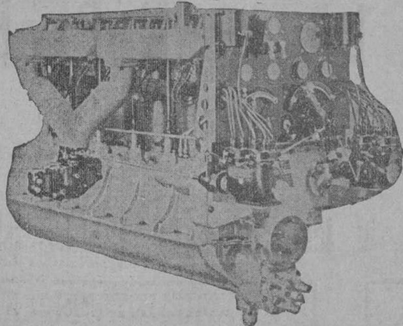
Uno de los seis motores Packard que constituyen la fuerte motorización del dirigible Shenandoah, con un total de 1,800 caballos de fuerza.
