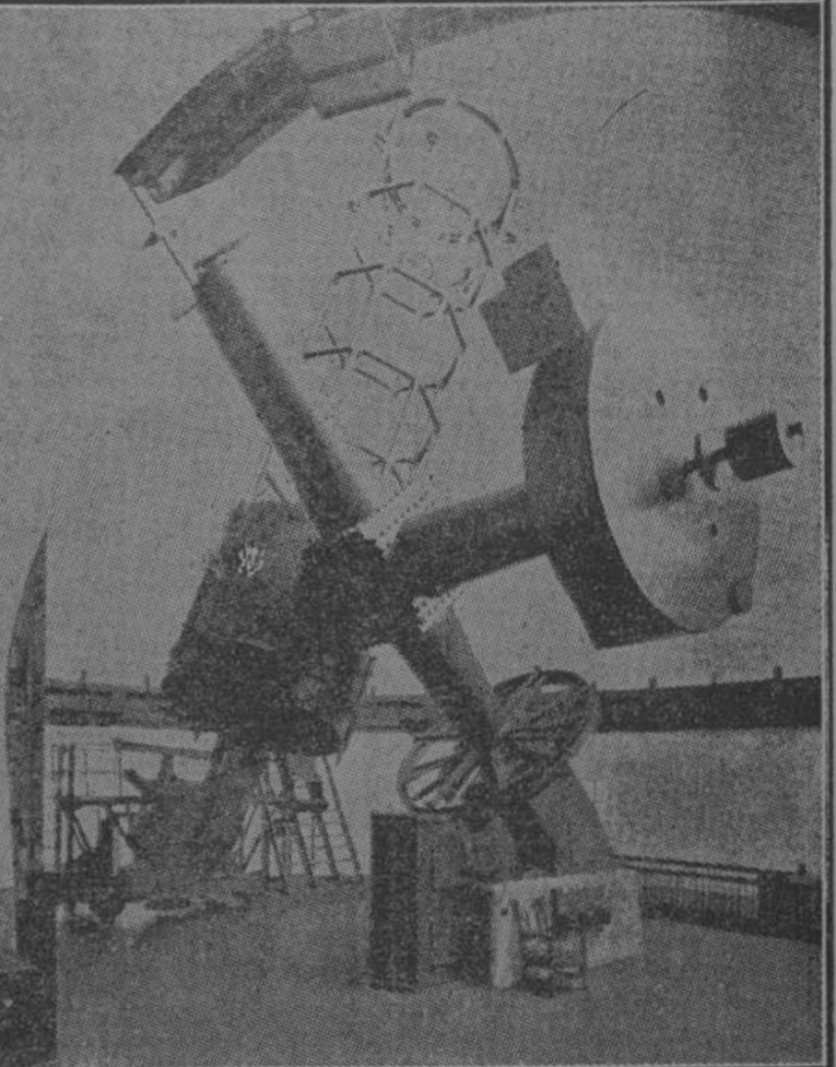
El reflector de 72 pulgadas con el espectróscopo agregado.
