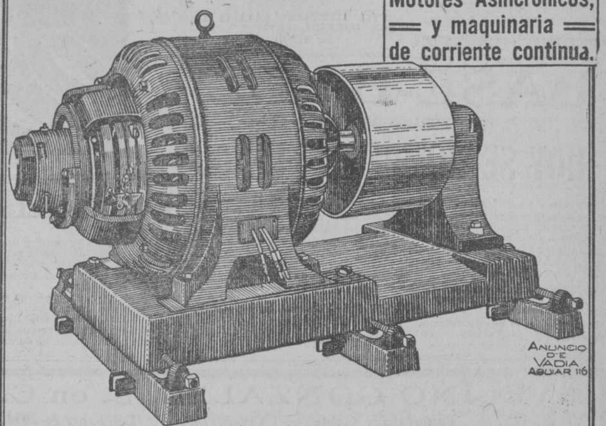
Motor trifásico tipo "AV" 440 volts, 60 períodos y 600 revoluciones por minuto 100 H. P. IDEAL PARA CENTRIFUGAS
