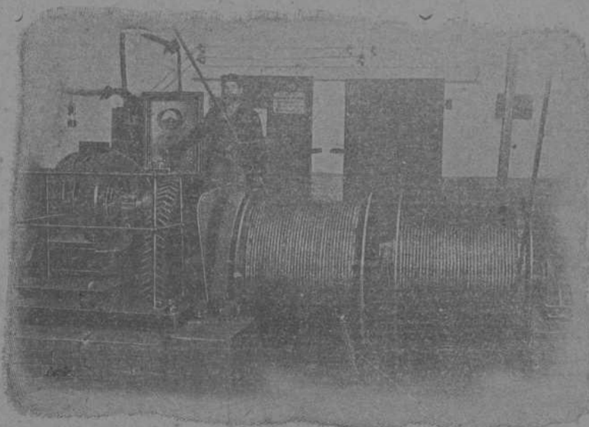
Torno doble para minas, movido por un motor de corriente alterna tri'ásica
