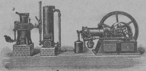
Gasógeno DEUTZ para Gas pobre
