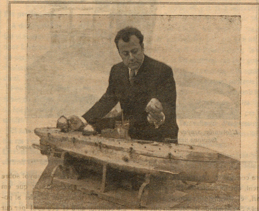
El senyor Cosme Salomó demostra pràcticament la instal·lació de seu invent—que permetrà la salvació de la tripulació dels submarins—i l'emplaçament de les boies salvavides en el casc del submarí.
