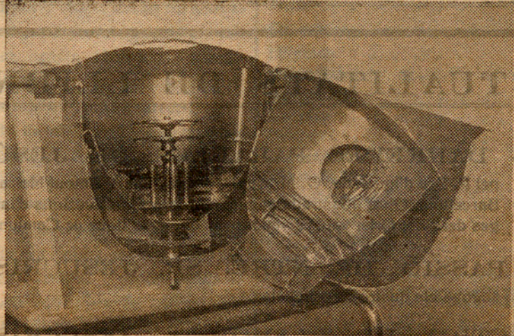
Interior d'una de les boies inventades pel senyor Salomó, en la qual pot observar-se el mecanisme descrit en aquest reportatge. Cal observar la contra-boia o alveolo, a la part externa i que forma part del submarí.
