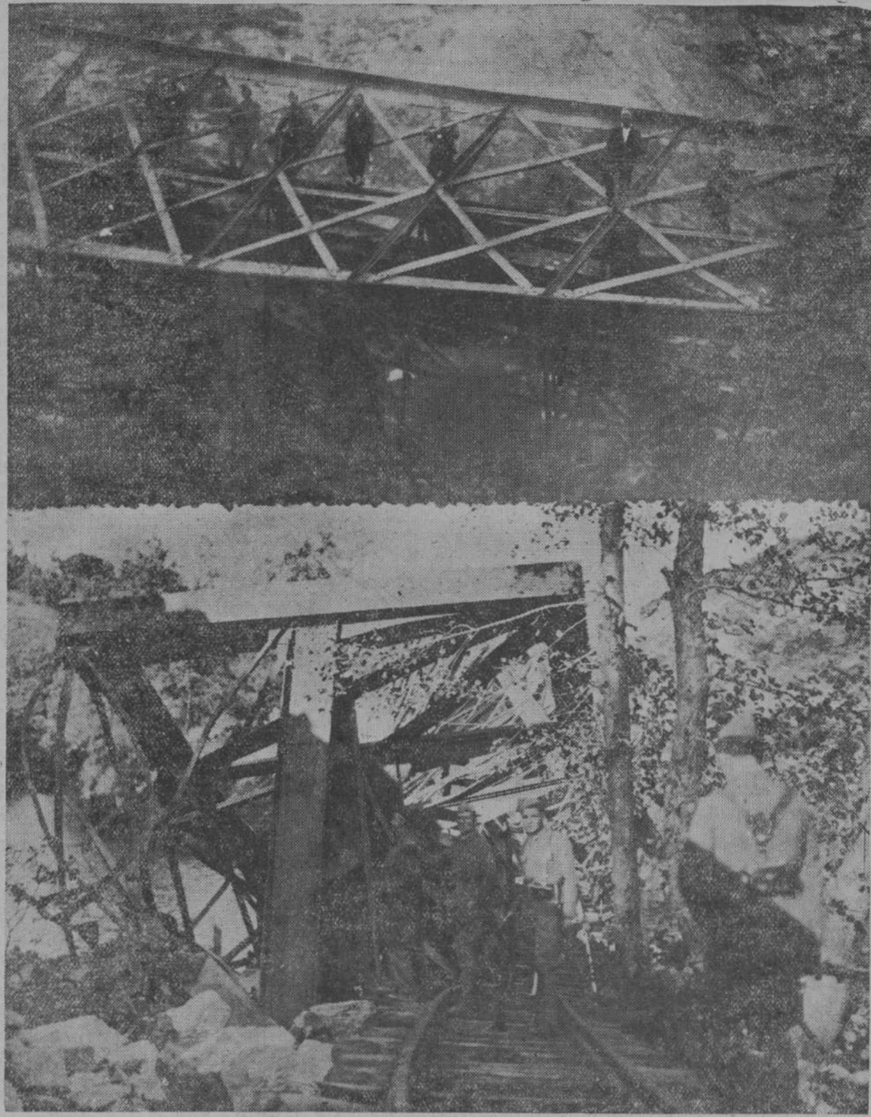
DE LOS PASADOS SUCECOS.—Dos aspectos del estado en que quedó el puente del Pedrón, del ferrocarril de La Robla, en Arroyo (Reinos), volado por los rebeldes. (Fotos obtenidas por el distinguido aficionado Sr. Ferret.)
