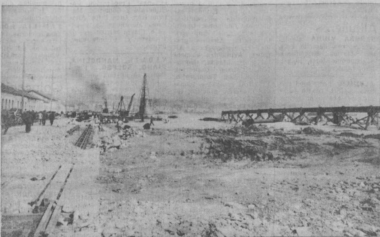
Avanzan las obras de los nuevos muelles. La parte de relleno gana cada día unos metros al mar. Un impulso más y el puerto de Santander dispondrá de una nueva y excelente zona de servicios para su tráfico. (Fot. Alejandro.)
