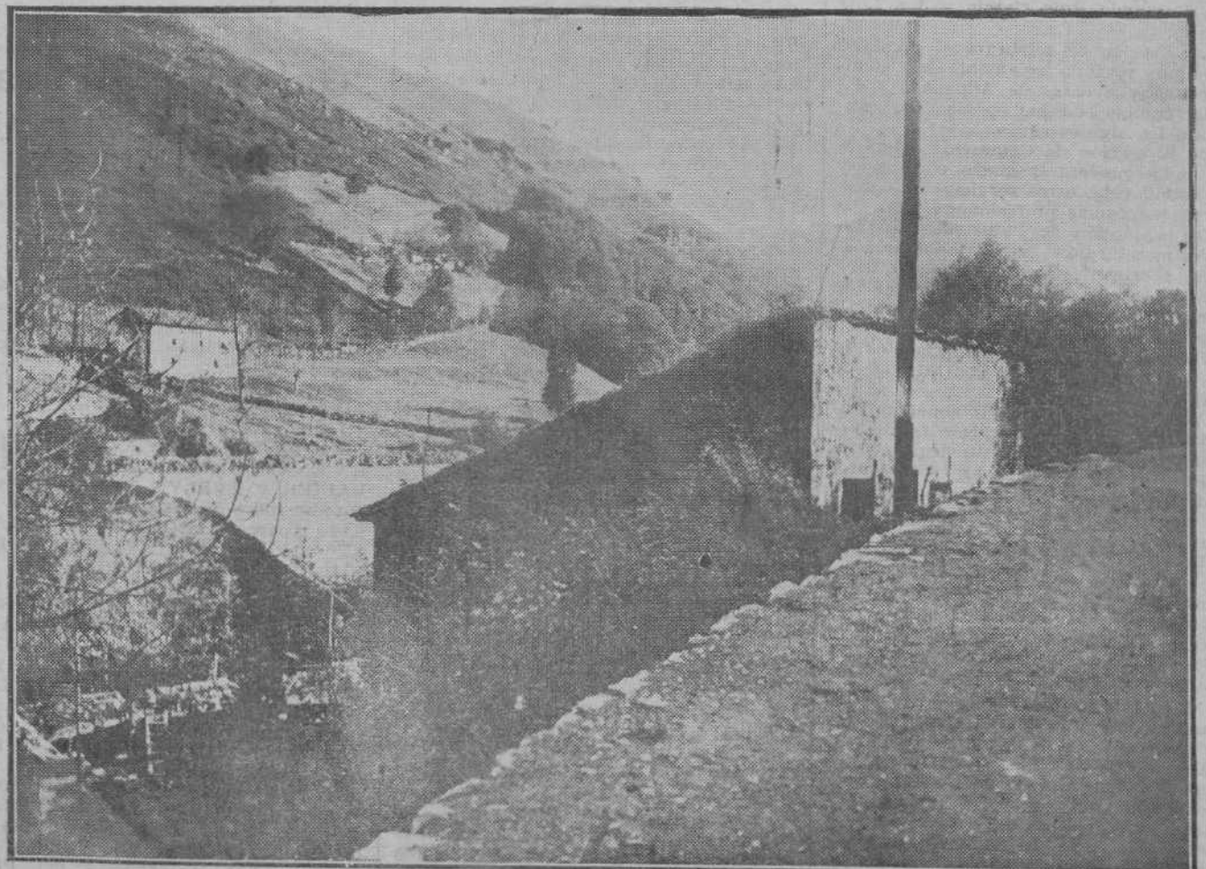
SAN MIGUEL DE LUENA.—He aquí el profundo valle que ha de atravesar, sobre un gigantesco viaducto, el ferrocarril Santander-Mediterráneo. García Alvarez ha obtenido la foto, sin indicación previa, desde el mismo lugar donde el señor Martínez de Velasco concibió la solución de esta interesantísima parte de su proyecto.
