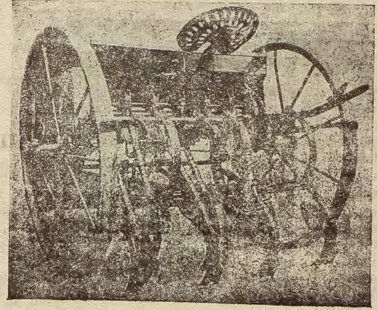
Sembradora RUD SACK
