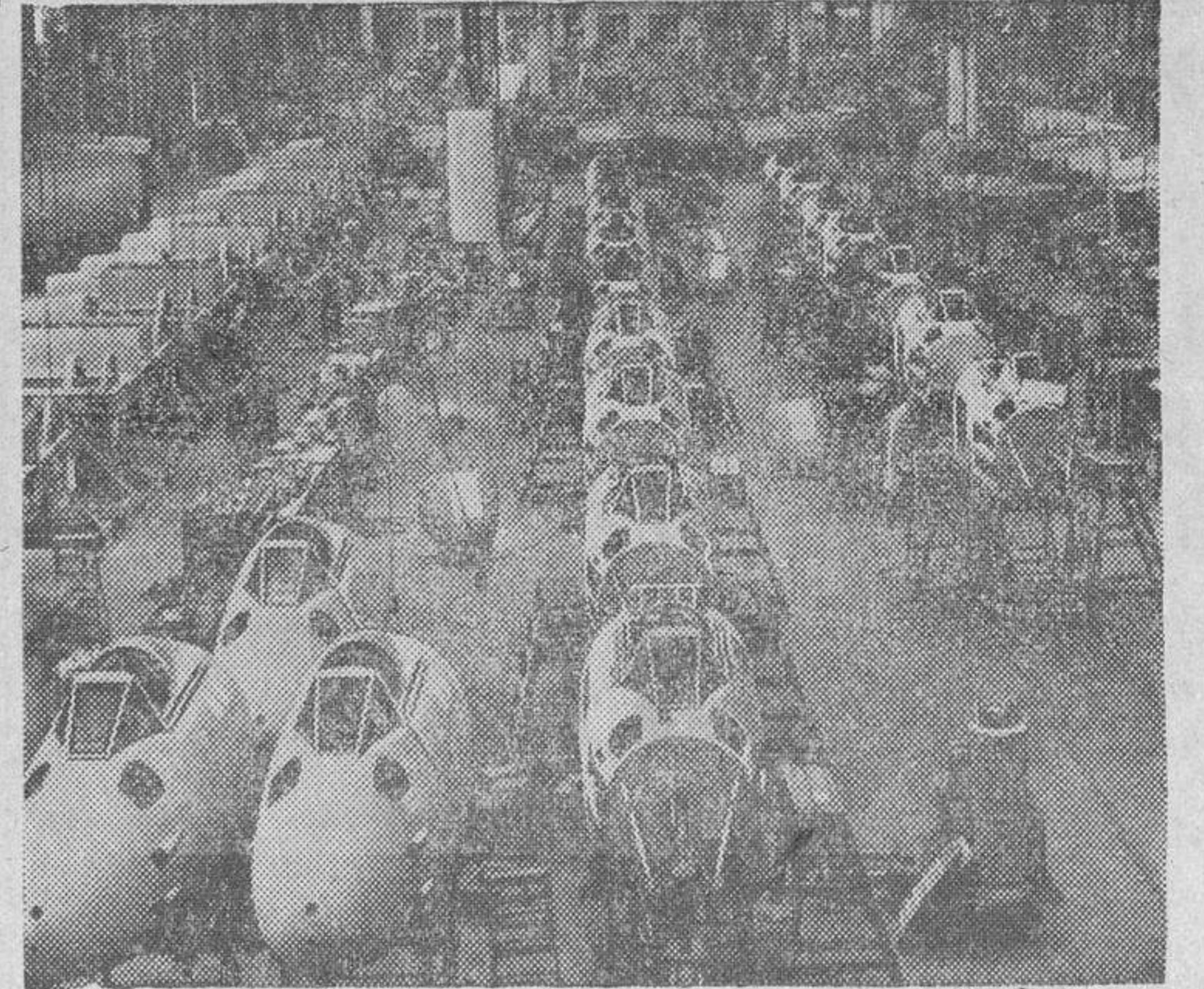
Con la perfección del motor de chorro de gases, por el Comodoro del Aire británico, sir Frank Whittle, se abrieron nuevos horizontes para la aviación. En esta fotografía podemos ver los «Ghost Meteor IV», en construcción, en los talleres de la Gloucester Aircraft Company. (Foto Calpe).
