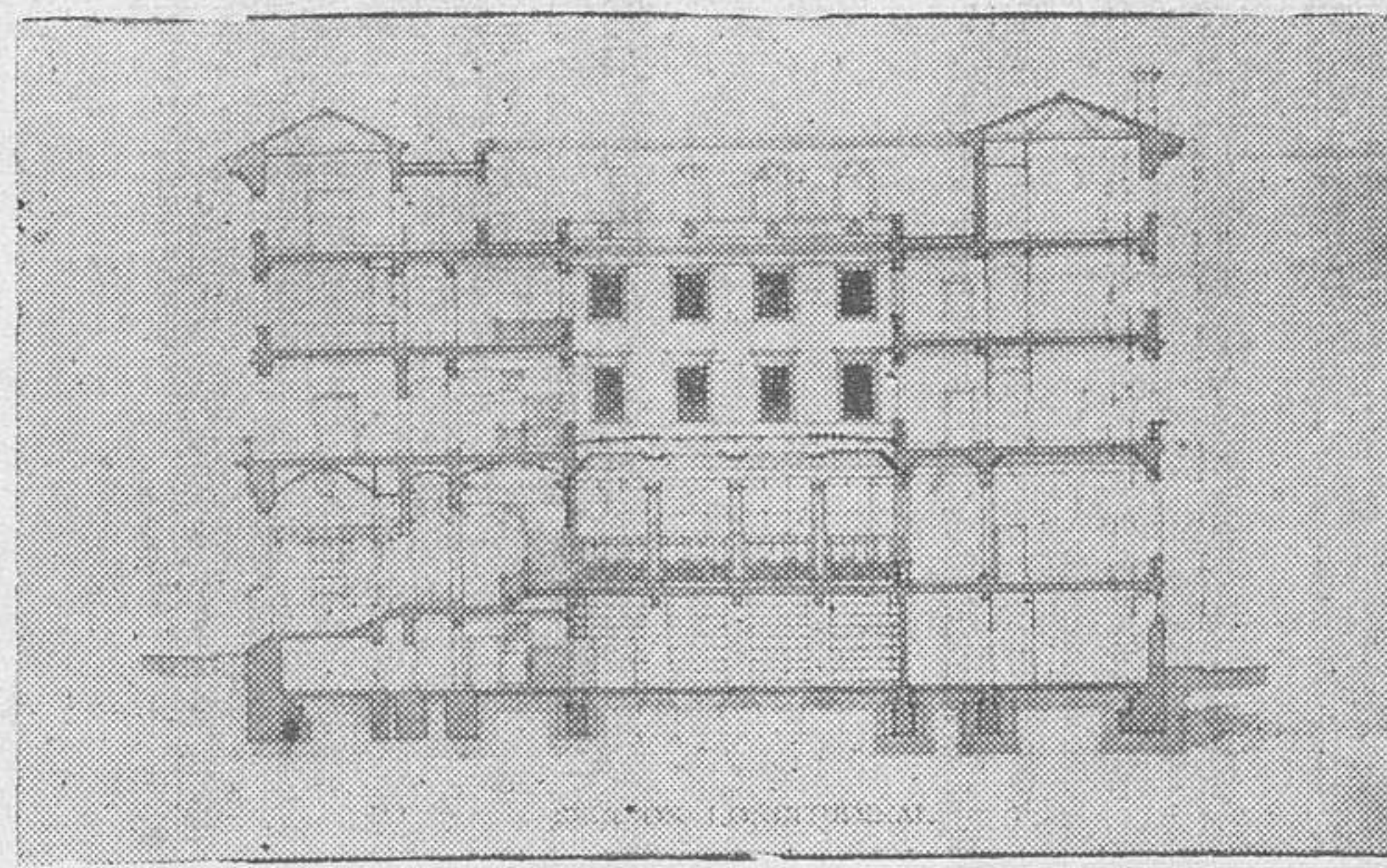
Sección longitudinal de la nueva Delegación de Hacienda, en el que pueden apreciarse los diversos pisos, estructura del patio, archivo y zaguán.
