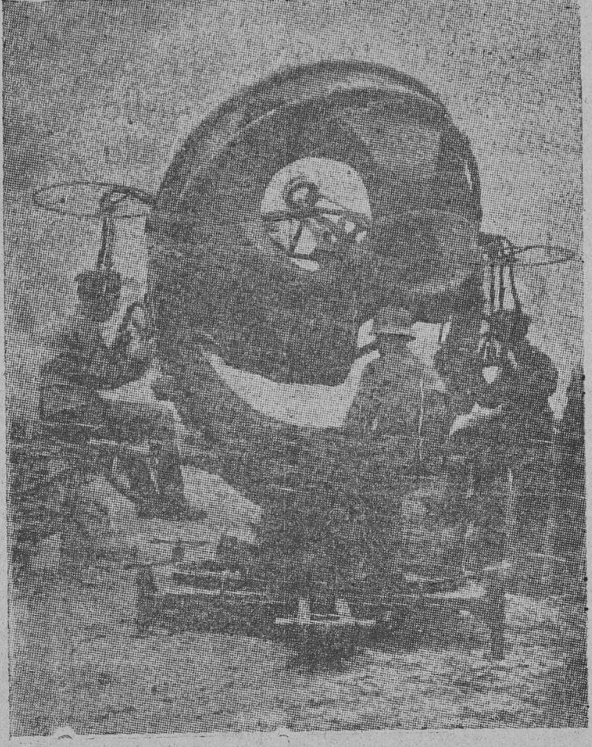
Detector de sonidos. Millares como éste, en torno a Berlín, avisan la llegada del enemigo aéreo. Cualquier ruido de motor es registrado a la distancia de 100 kilómetros. En el pequeño anillo central, que es como el foco de un espejo parabólico, son recogidos los ruidos y lanzados a las paredes interiores a las que están aplicados micrófonos que le amplifican; dos soldados los escuchan como médicos auscultadores. Todo el aparato gira alrededor de su eje vertical; además el "espejo" auditivo puede inclinarse más o menos, en forma que se pueda orientar hasta conseguir la mayor intensidad de sonido e indicar de esta manera el lugar de donde éste procede
