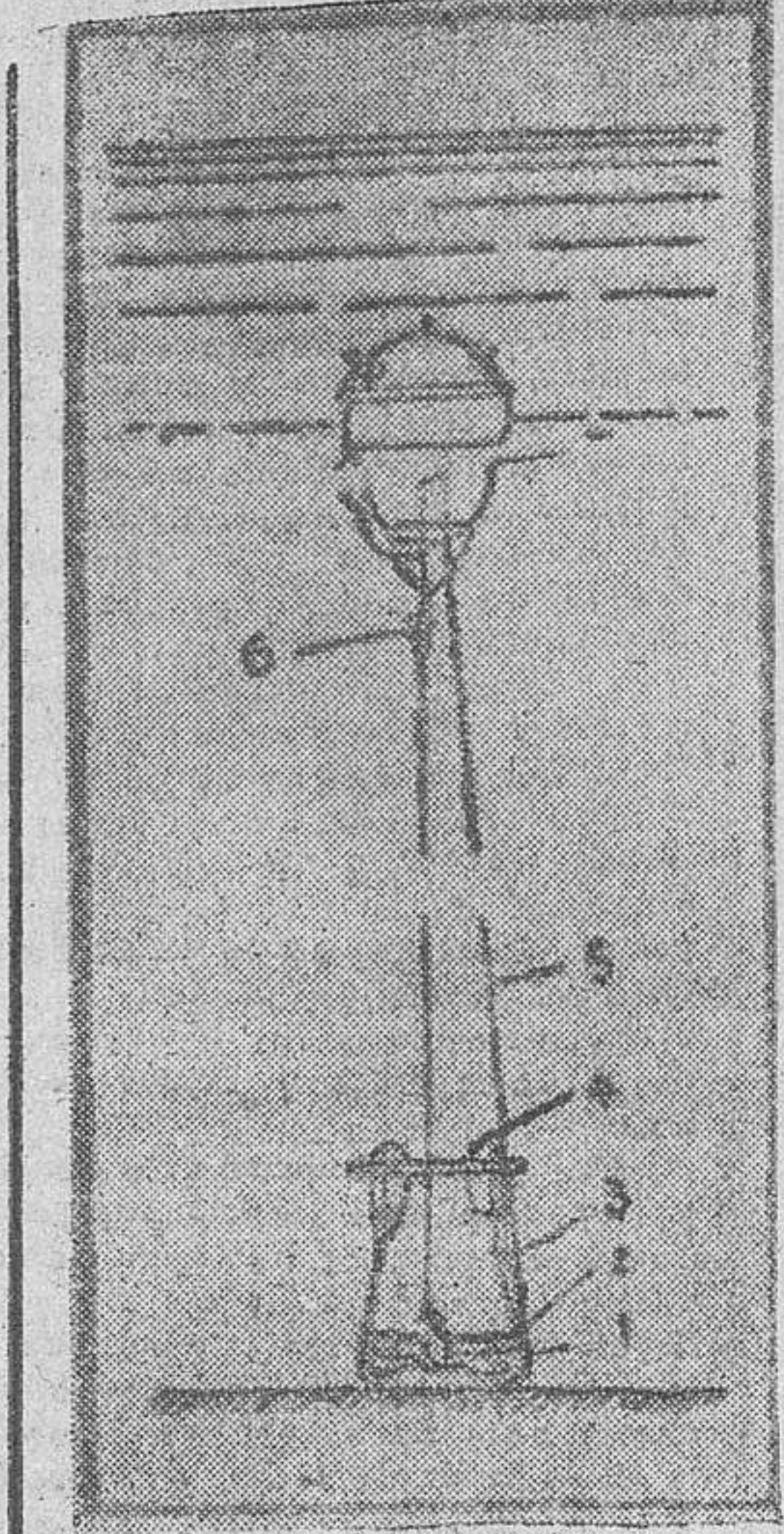
Esquema de una mina
