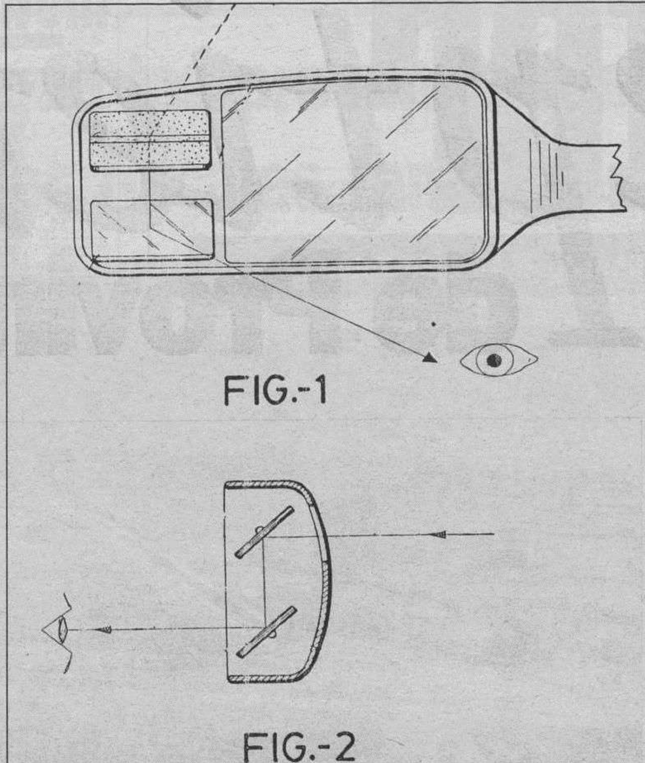
Con los dos espejos pequeños y la apertura en la carcasa del retrovisor es posible ver los vehículos ocultos por un camión.
