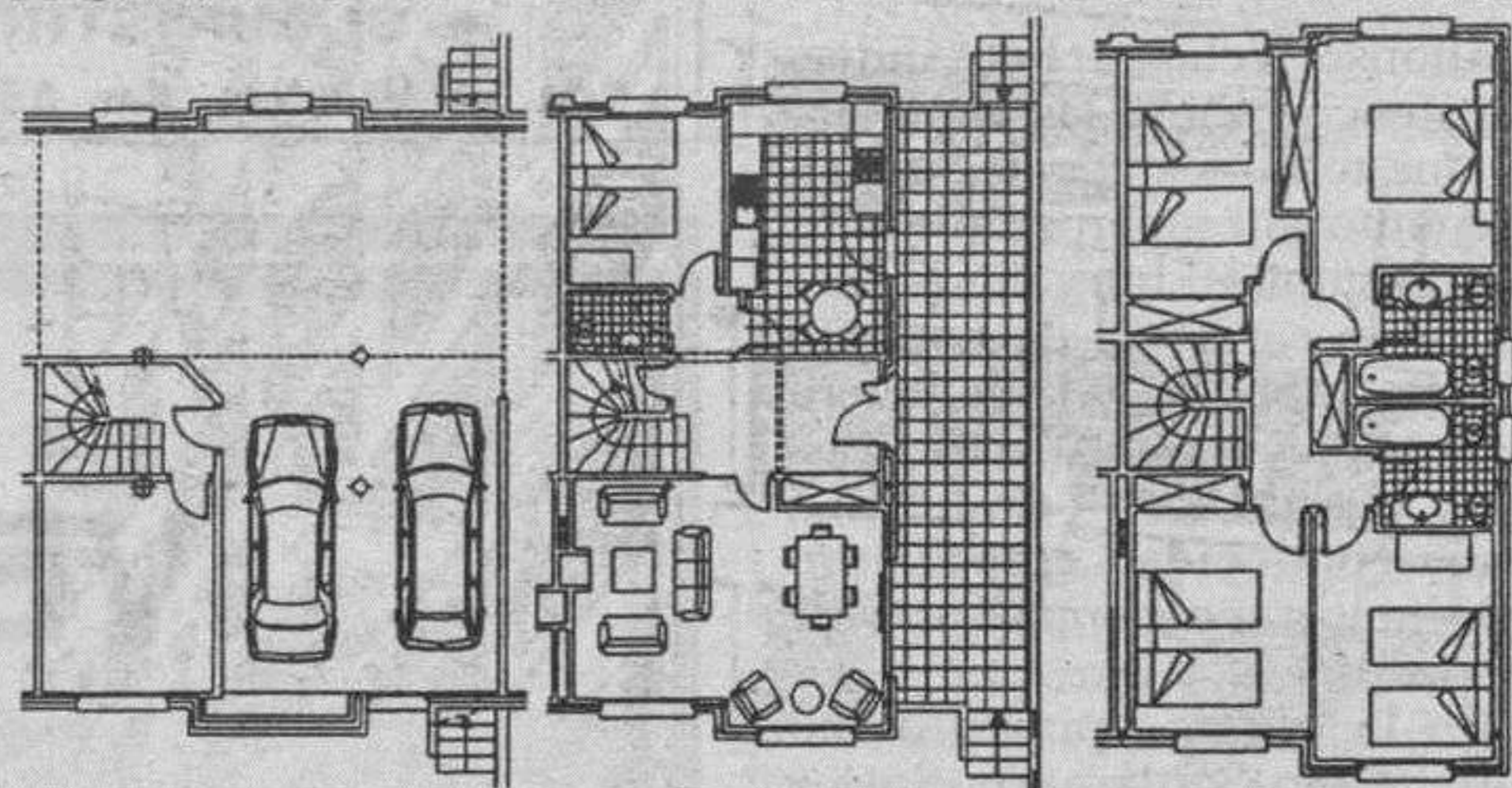
PLANTA SOTANO PLANTA BAJA PLANTA PRIMERA
